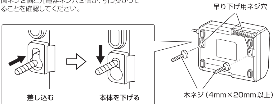
【充電器裏側】
