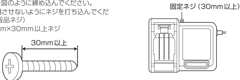
【充電器表側】
