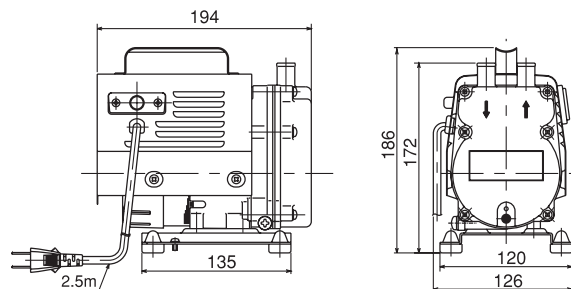
HP-50
