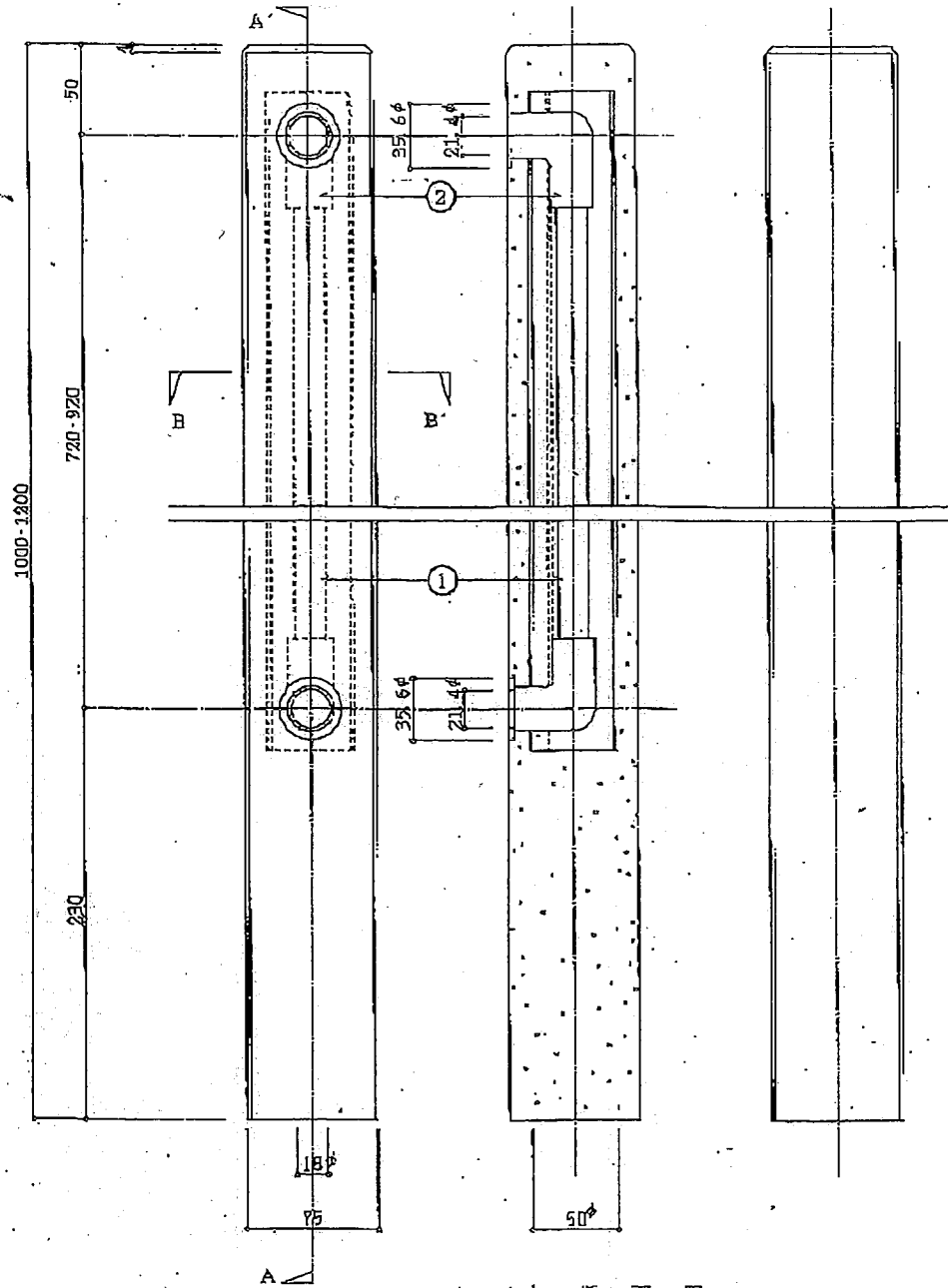
A-A 断面図
