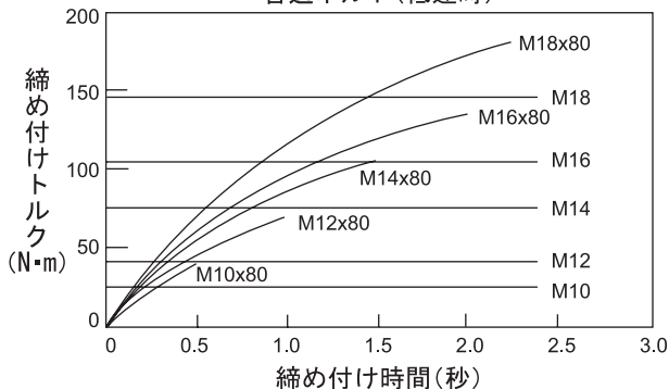
普通ボルト (低速時)
