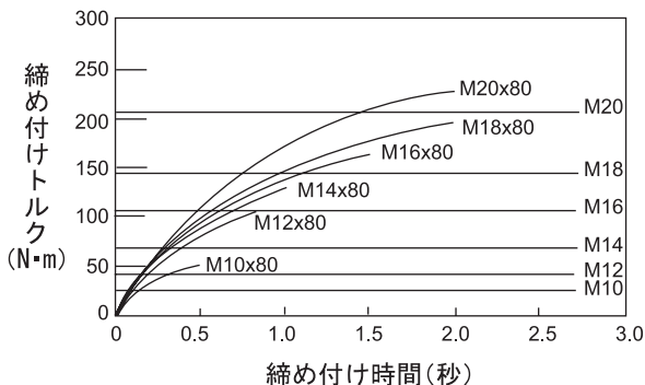
普通ボルト (低速時)
