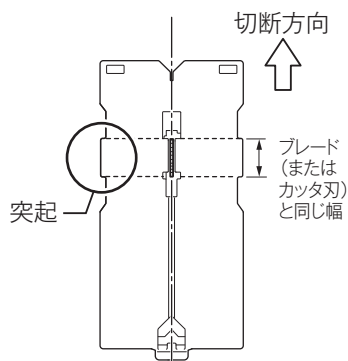
ベースカバーをブレード（またはカッタ刃）側から見た正面図
