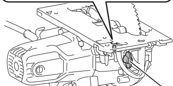
角度調整用ツマミネジ（前後2か所）
