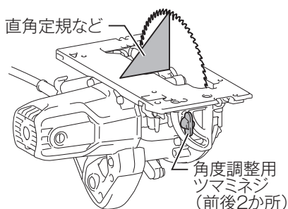
角度調整用ツマミネジ（前後2か所）
