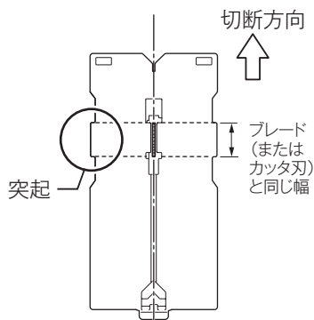
ベースカバーをブレード（またはカッタ刃）側から見た正面図
