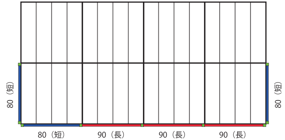
③フェンス6枚A
