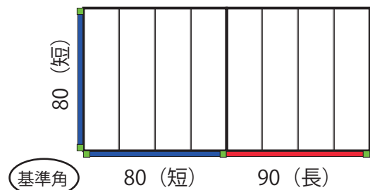
②フェンス 2 枚
