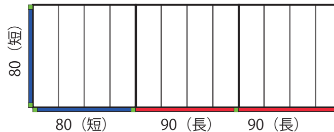
③フェンス 3 枚
