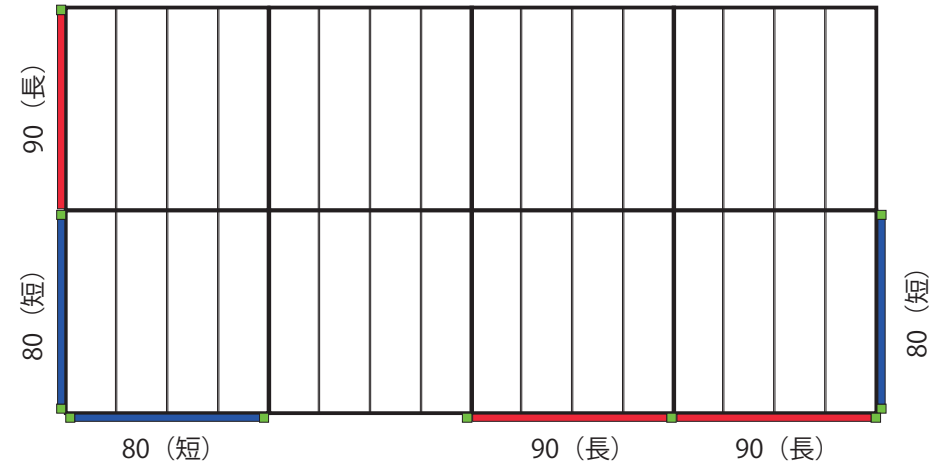
④フェンス6枚B
