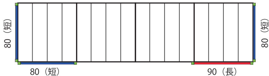
③フェンス 4 枚 A
