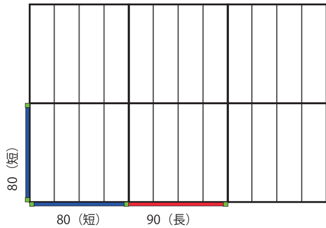
⑨フェンス 3 枚 B
