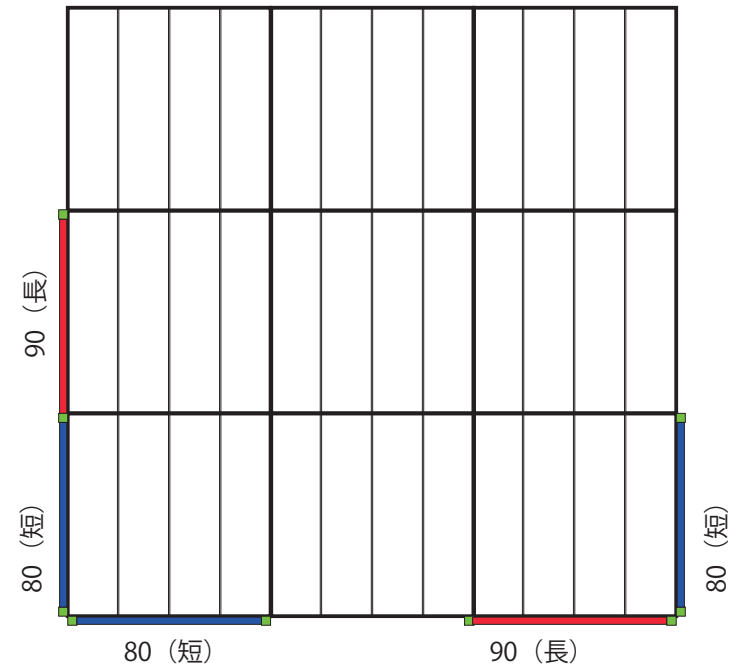
⑫フェンス 5 枚 D
