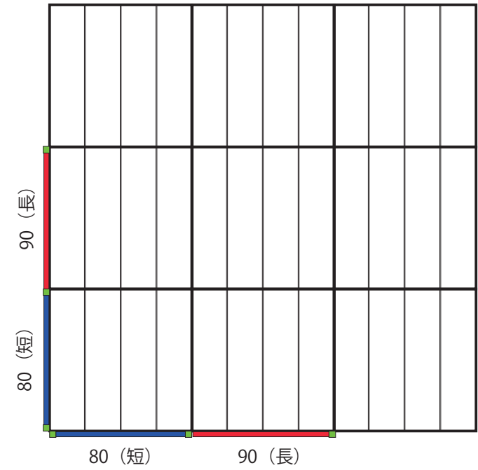
⑮フェンス 4 枚 C
