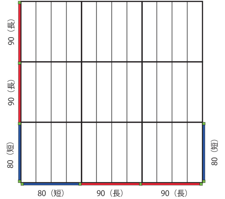
③フェンス 7 枚 A
