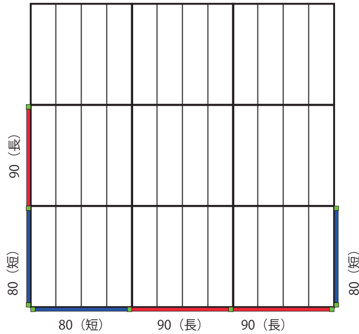
⑥フェンス6枚A
