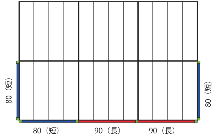
③フェンス 5 枚 A
