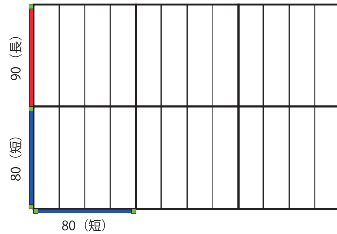
⑧フェンス 3 枚 A
