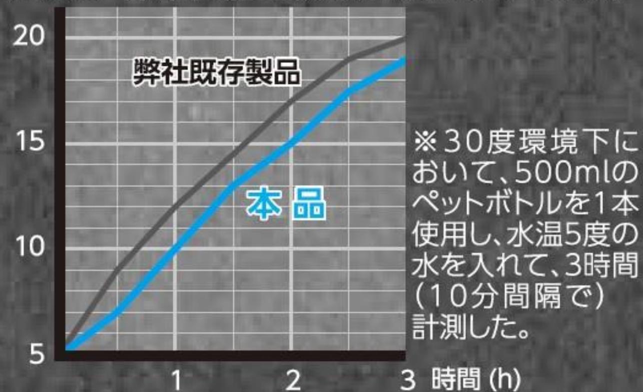
温度(℃) 保冷性能比較 (弊社既存製品との比較)
