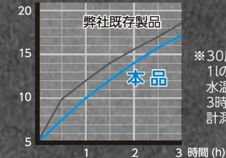
温度(°C) 保冷性能比較 (弊社既存製品との比較)
