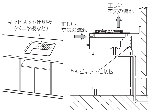
キャビネット仕切板設置例
