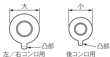
バーナーキャップ
