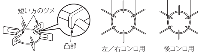
バーナーキャップ
