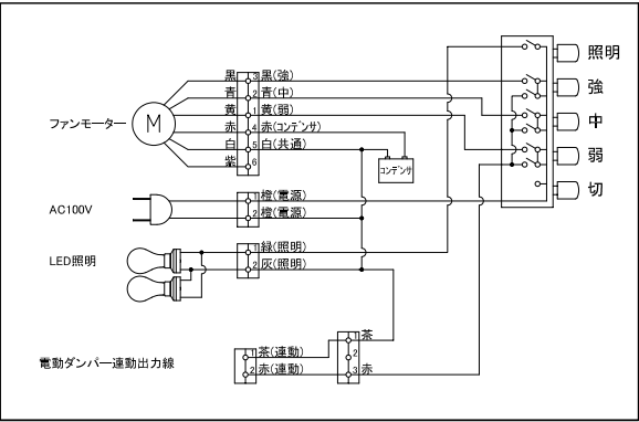
□結線図
