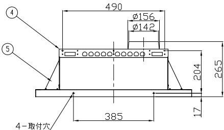
背面取付図
