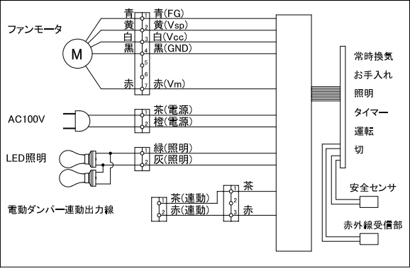
□結線図
