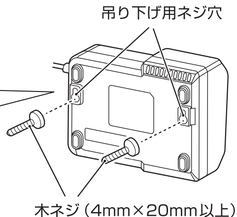
【充電器裏側】
