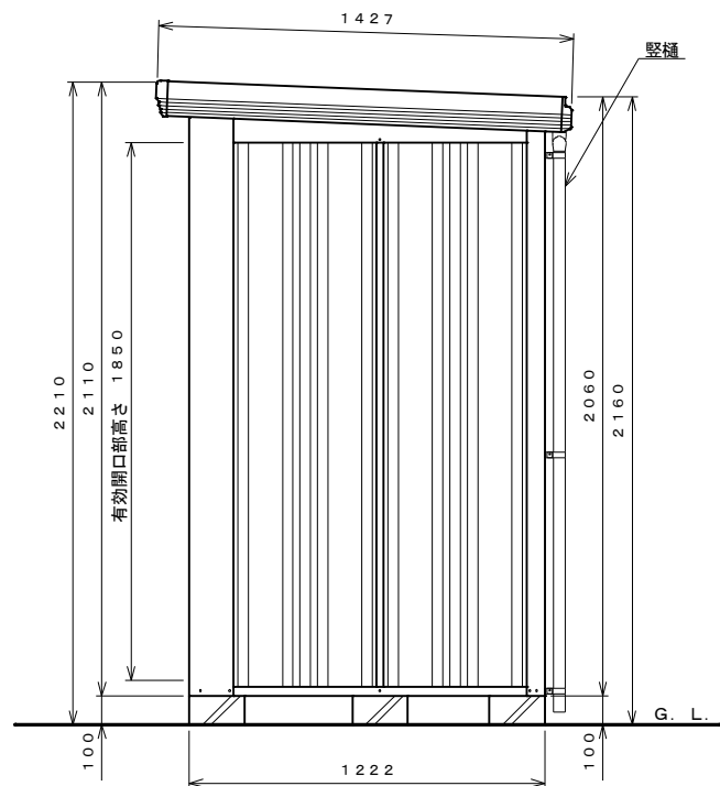
側面図 S=1:20
