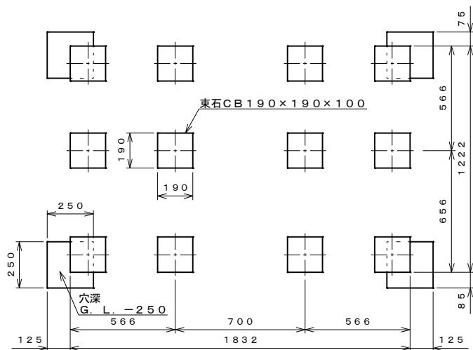
基礎伏せ図 S=1:20
