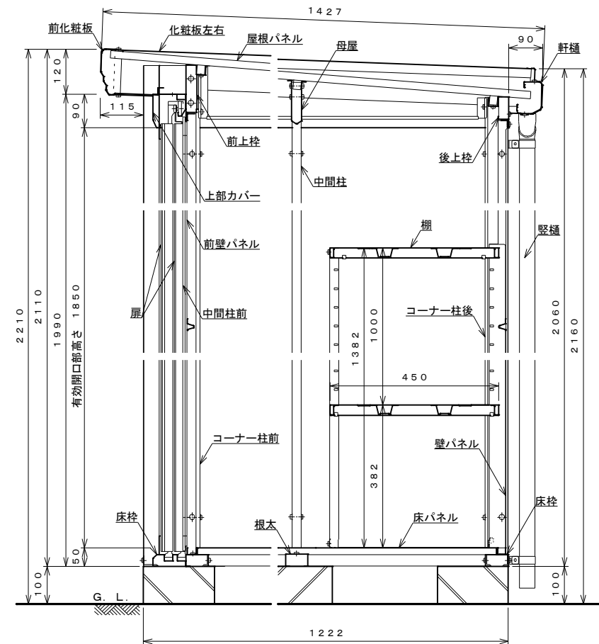
側面断面図 S=1:10
