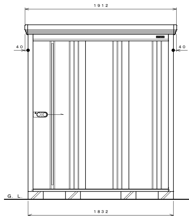
正面図 S=1:20
