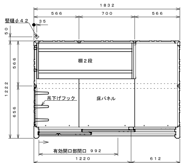
平面図 S=1:20
