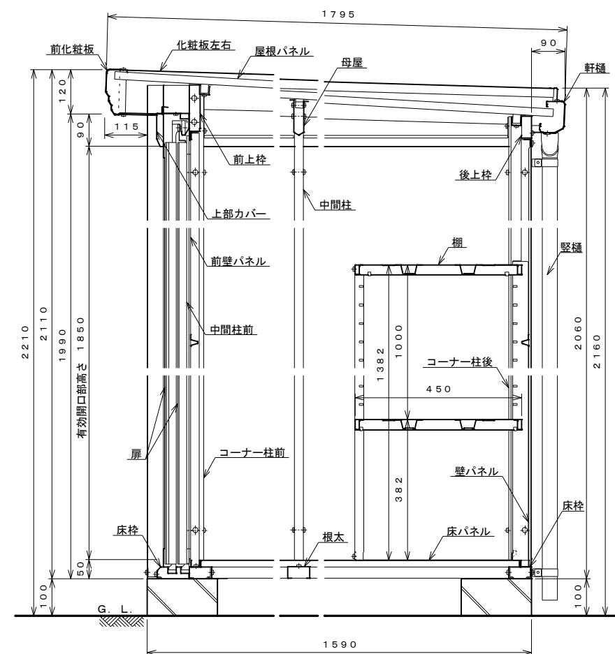
側面断面図 S=1:10
