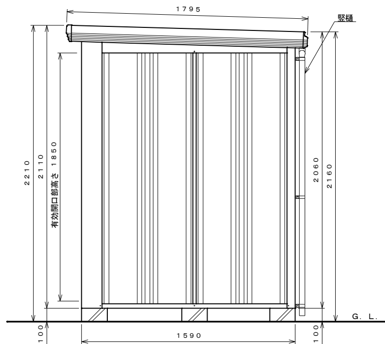
側面図 S=1:20
