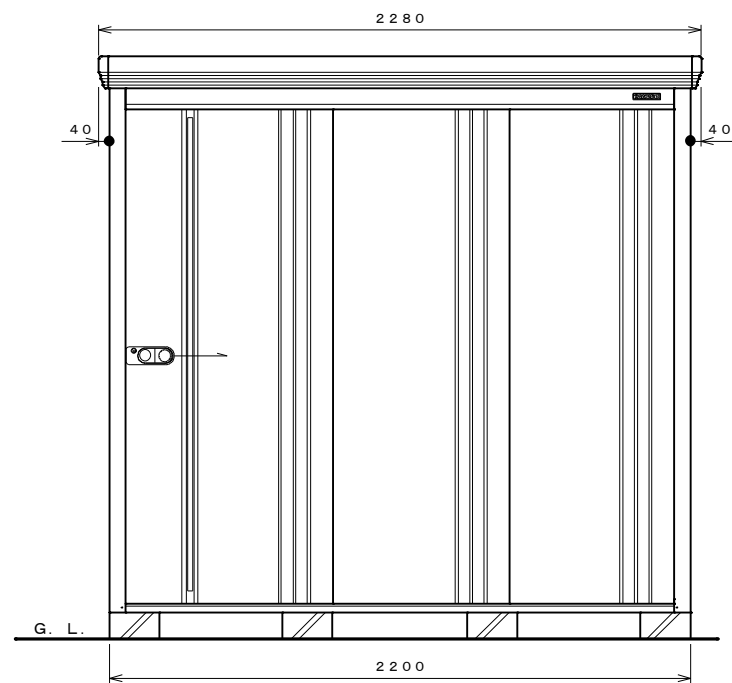
正面図 S=1:20
