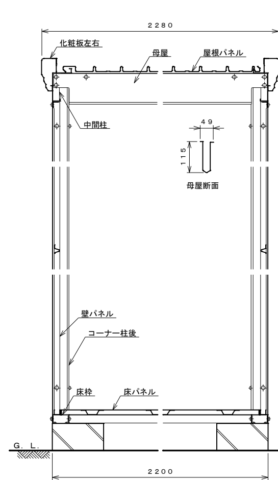
正面断面図 S=1:10
