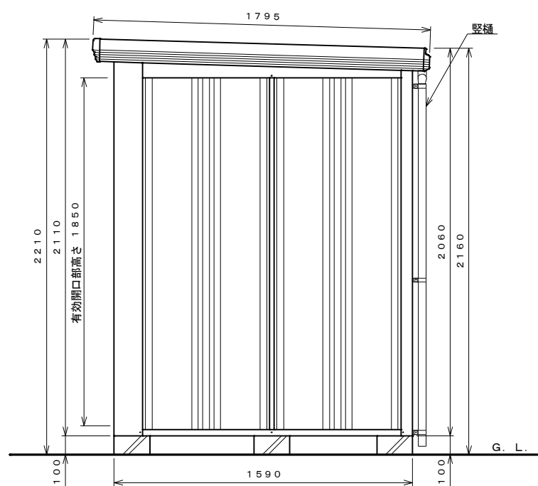
側面図 S=1:20
