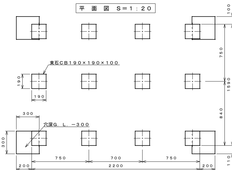
基礎伏せ図 S=1:20
