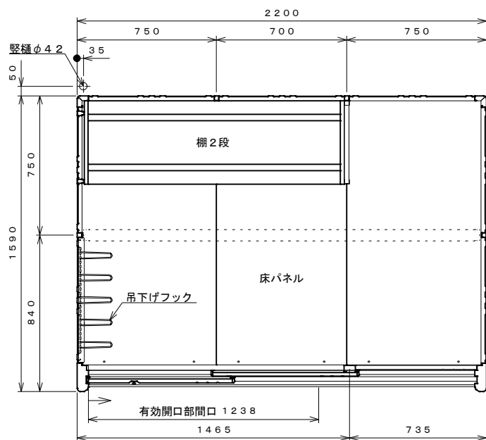
平面図 S=1:20
