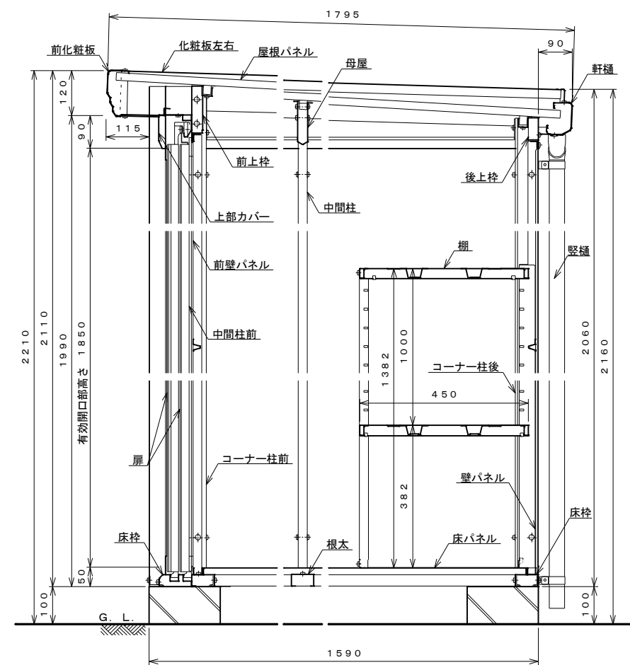
側面断面図 S=1:10
