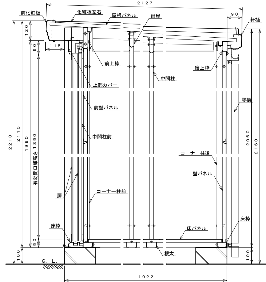
側面断面図 S=1:10
