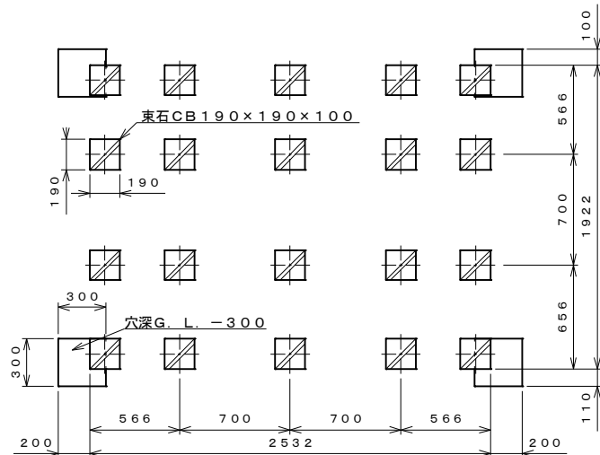
基礎伏せ図 S=1:30
