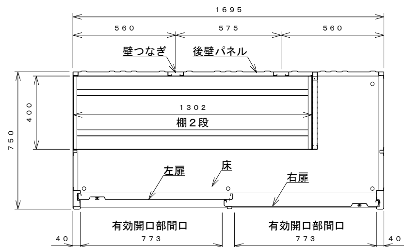
平面断面図
