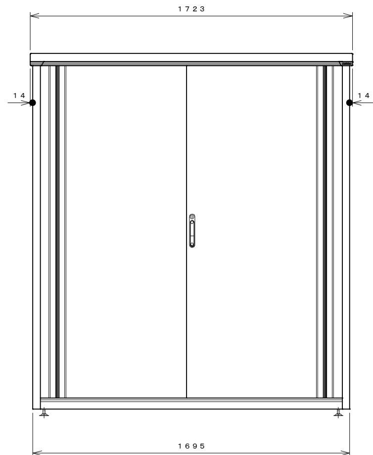
正面図
