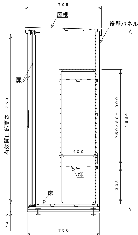
側面断面図
