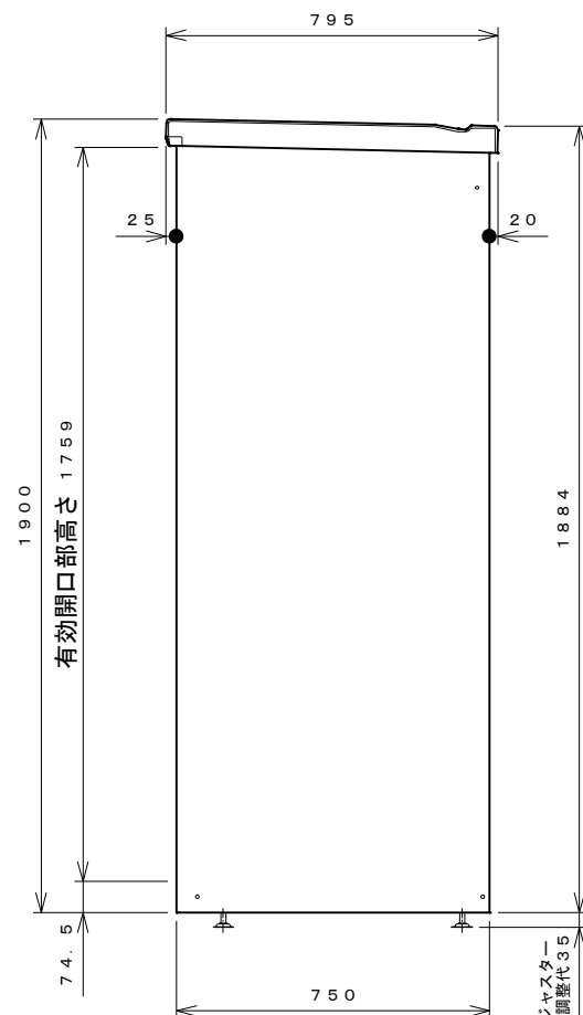
右側面図
