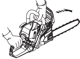
チェーンブレーキ作動
