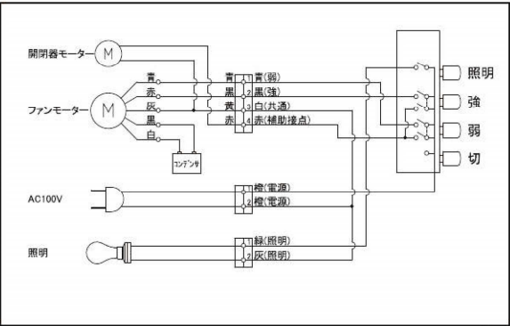
□結線図
