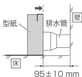
横から見た図
