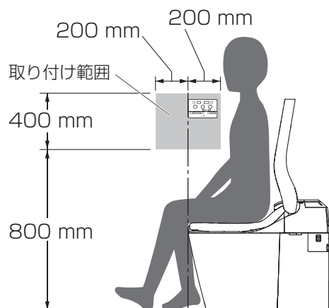
取付位置の目安
