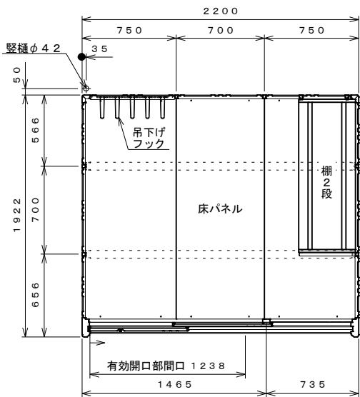
平面図 S=1:30
