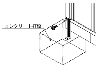
アンカー要領図
