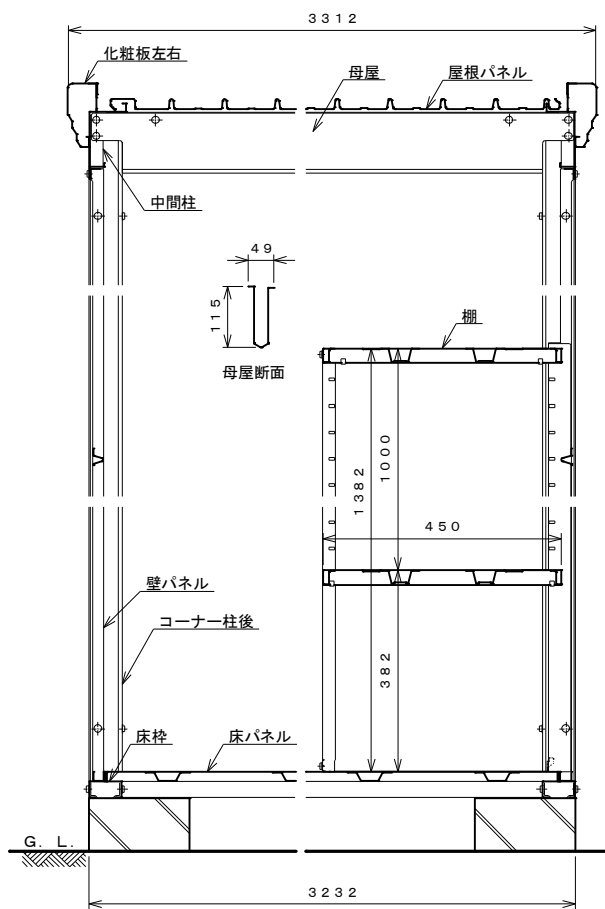
正面断面図 S=1:10
