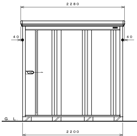
正面図 S=1:30
